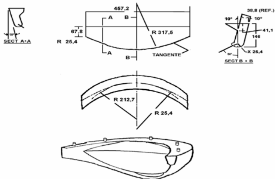
Figura 2.- Bloques metálicos patrón usados en la prueba de resistencia de la ceja al desmontaje del rin.
