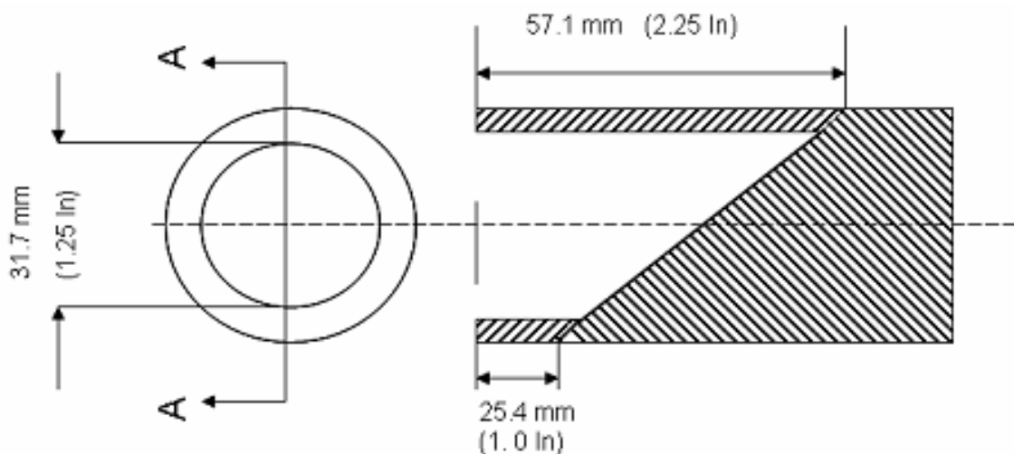
Figura 1. Cilindro para partes pequeñas
