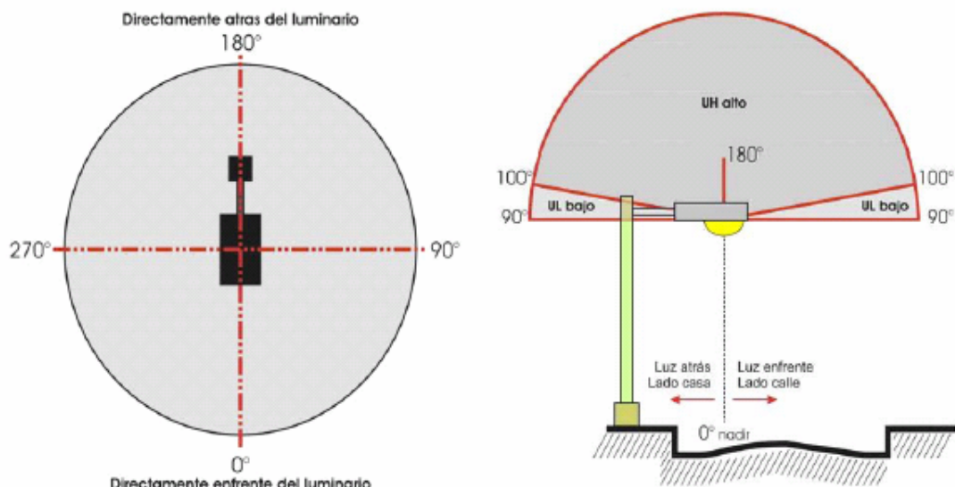
Figura D6. Angulos sólidos secundarios verticales para luz arriba
