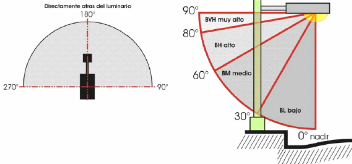
Figura D5. Angulos sólidos secundarios verticales para luz atrás o lado casa
