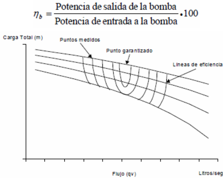
Figura 3.- Curva esquemática de capacidad vs carga total para la verificación de la eficiencia garantizada
