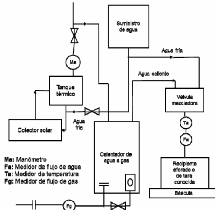
Figura A 1 - Esquema de instalación para medir el consumo de gas de un calentador de agua solar acoplado a un calentador de agua a gas, como respaldo.
