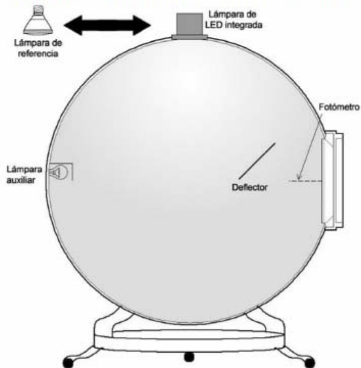
Figura K2 - Configuración de la esfera integradora 2 \pi
