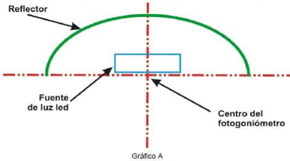
Figura D1. Montajes del luminario bajo prueba en el goni-fotómetro
