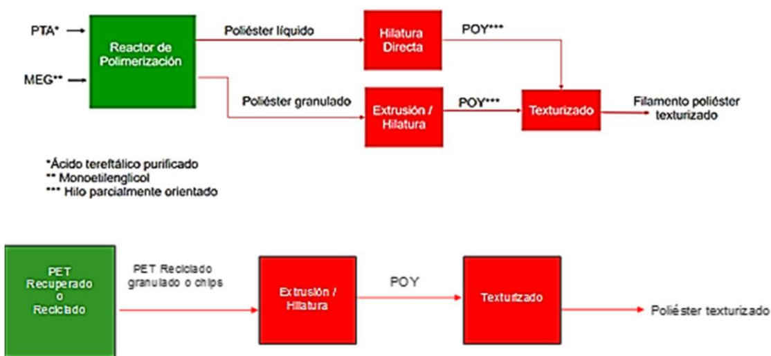
Diagrama del proceso productivo de PFTT
